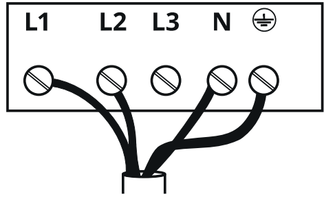
380V-415V 2N ~
