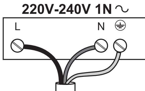
Pieslēguma shēma
