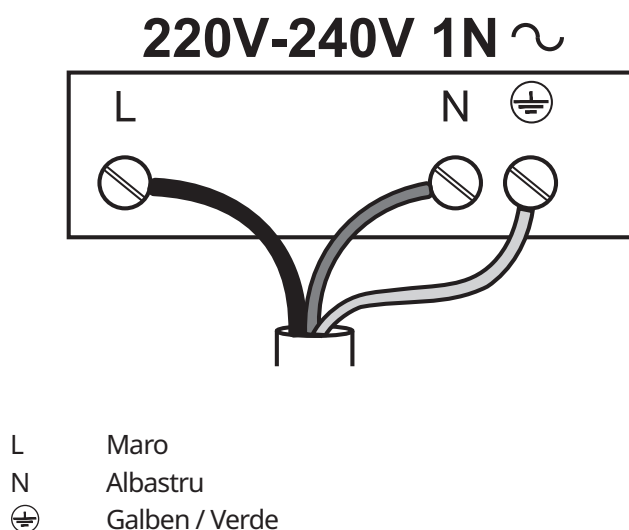
Schema de conexiune
