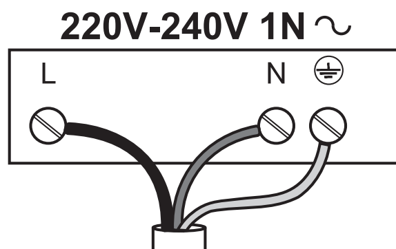
Схема на свързване
