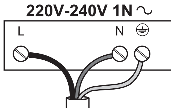
Tilslutningsdiagram
