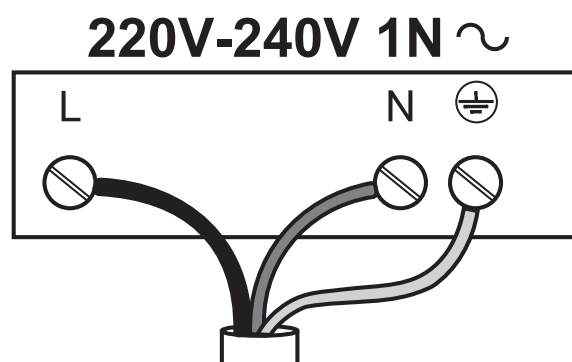
Shema za priključitev
