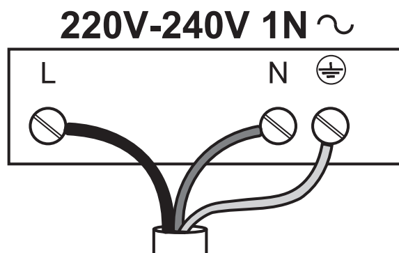
Схема на свързване
