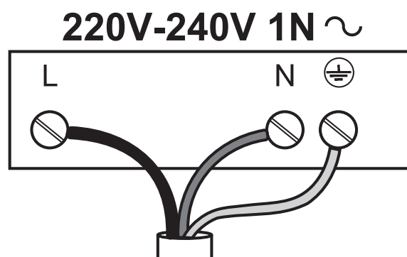
Schema de conexiune
