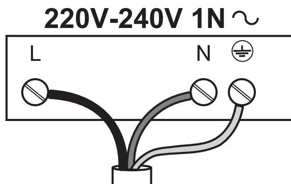
Schemat połączeń
