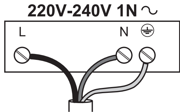
Схема підключення
