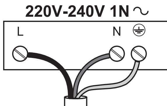
Schéma zapojenia
