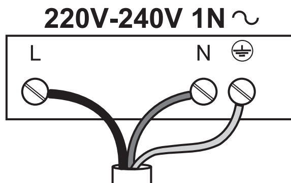
Kapcsolási rajz
