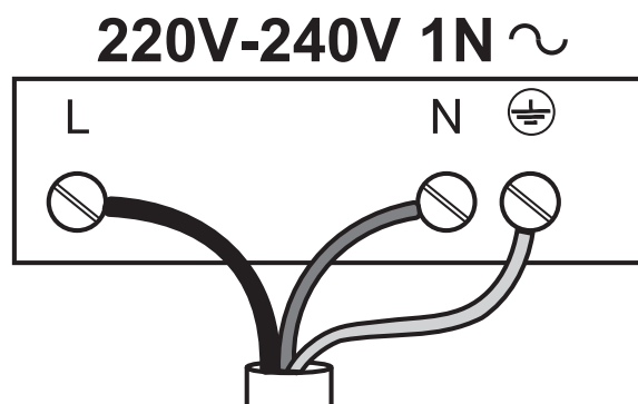
Esquema de conexión
