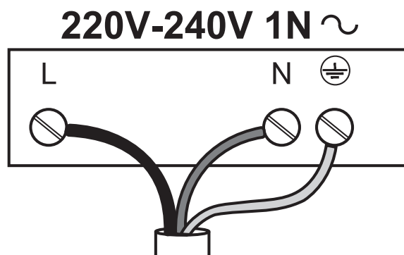
Pieslēguma shēma
